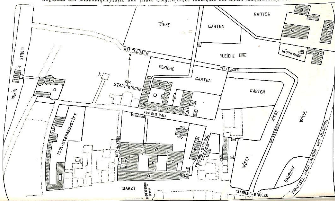
Lageplan des Diakonissenhauses und seiner Tochterhäuser innerhalb der Stadt Kaiserswerth, 1836—1903.
